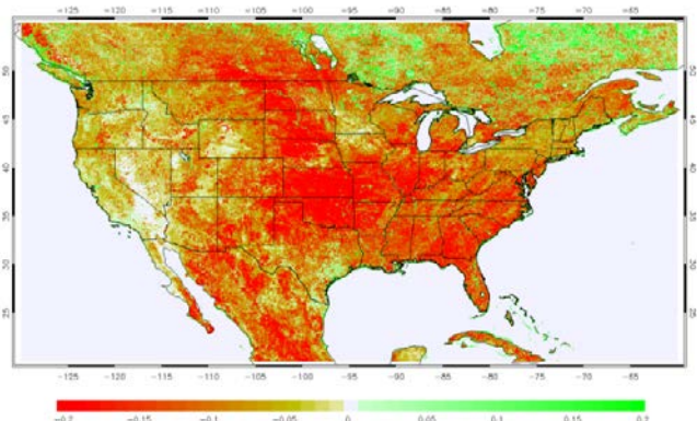
VIIRS GVF anomaly (15 August 2012)
